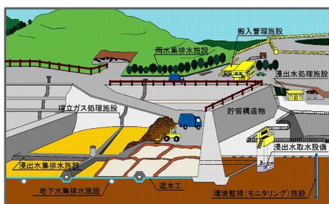
図 2.11 最終処分場施設の構成
