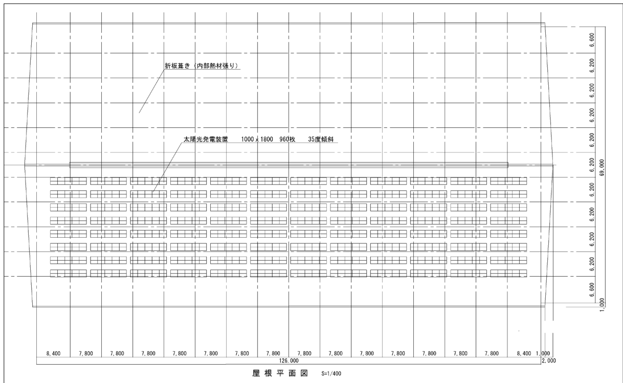
図 3.32 被覆施設屋根平面図
