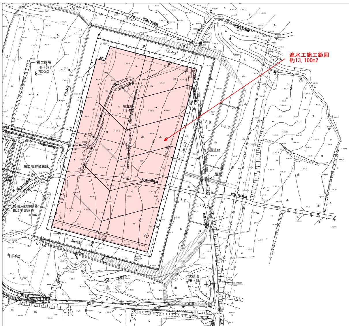
図 3.10 遮水工平面図
