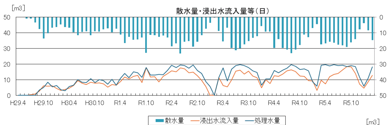
図 3.18 月別散水量、浸出水量日換算値実績の経時変化
