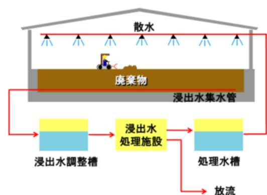
図 2.11 最終処分場施設の構成
