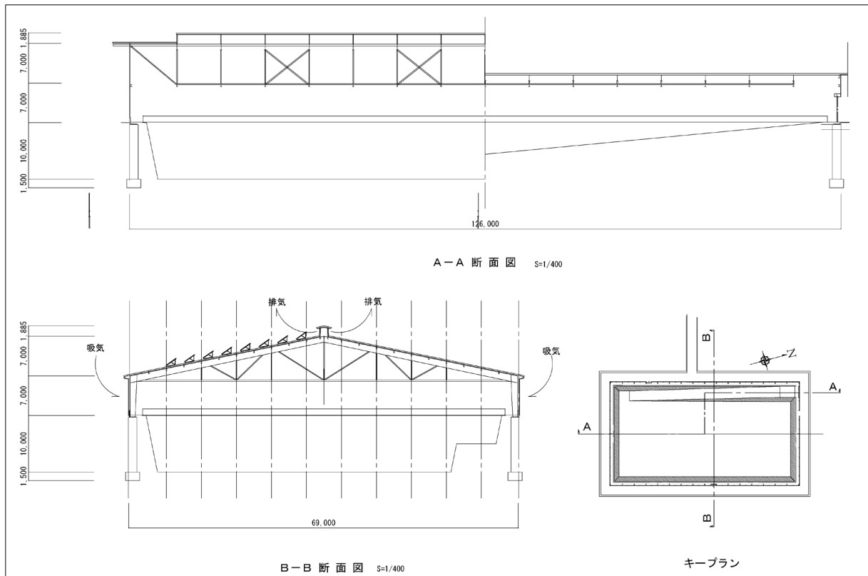
図 3.33 被覆施設各部断面図
