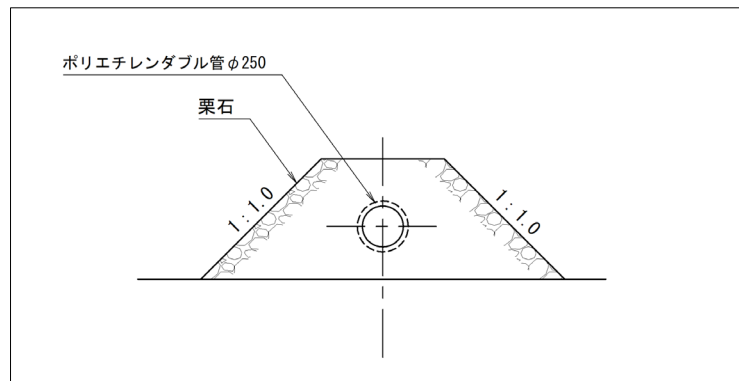
図 3.15 浸出水集排水施設（幹線）標準断面図
