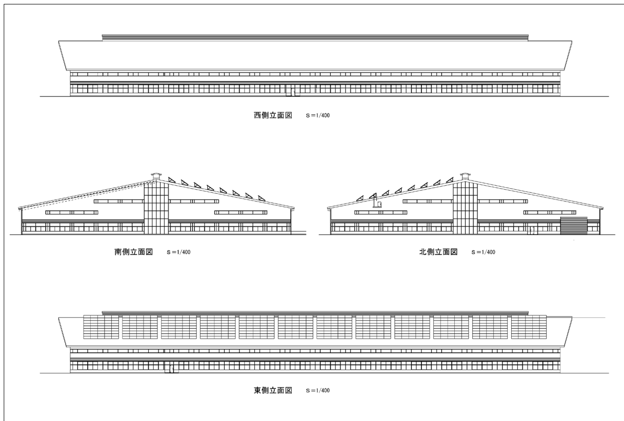
図 3.34 被覆施設立面図
