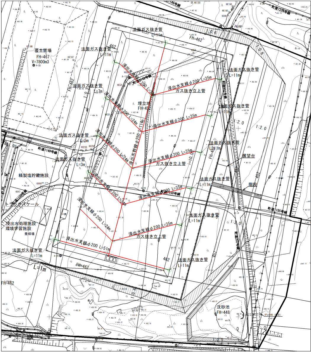
図 3.14 浸出水集排水施設平面図
