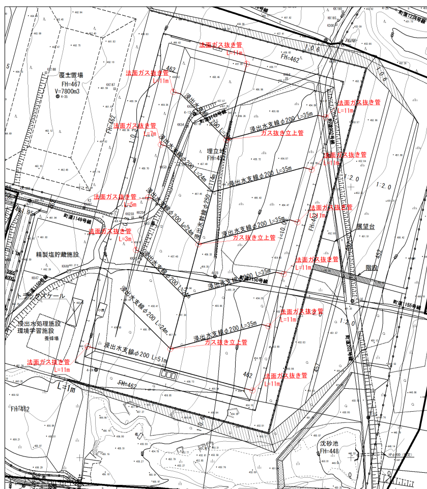
図 3.28 埋立ガス処理施設平面図
