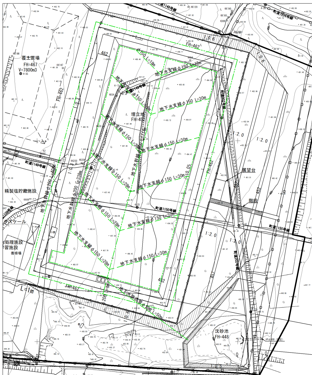
図 3.4 地下水集排水施設計画平面図
