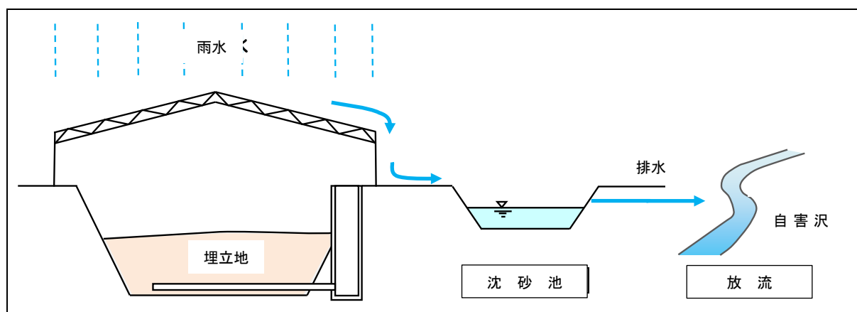
図 3.11 雨水集排水施設のイメージ図
