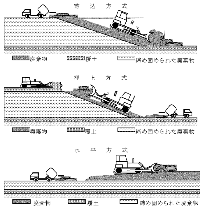
図 2.18 敷均し・転圧の方法
