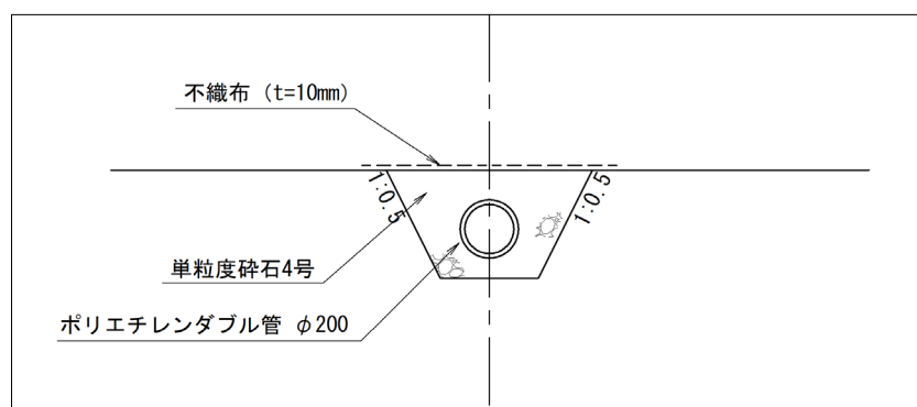
図 3.5 地下水集排水施設（幹線）標準断面図
