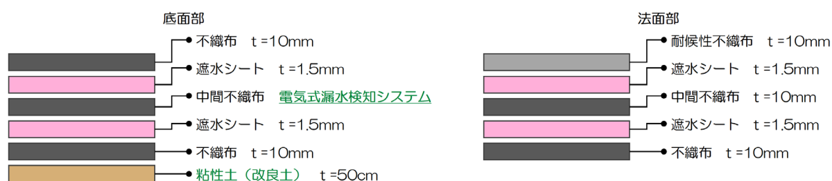
図 3.9 遮水工の構造（標準断面）
