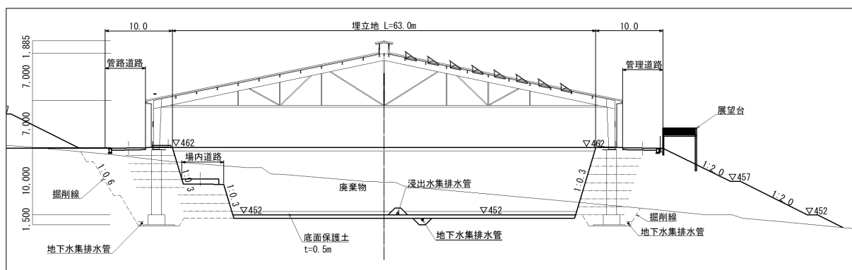
図 3.3 貯留構造物標準断面図
