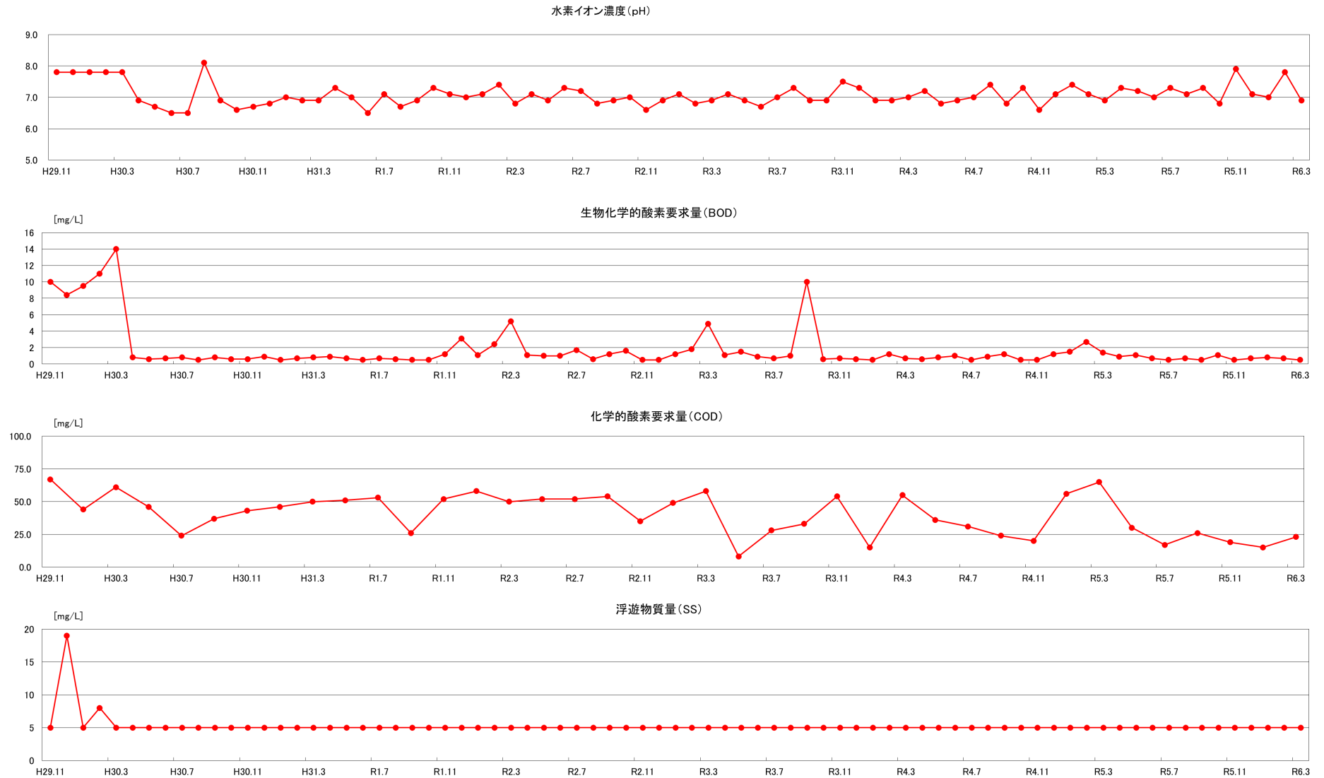
図 3.25 処理水水質の経時変化 (1/2)
