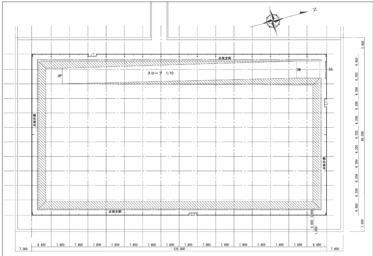
図 3.31 被覆施設 1 階平面図
