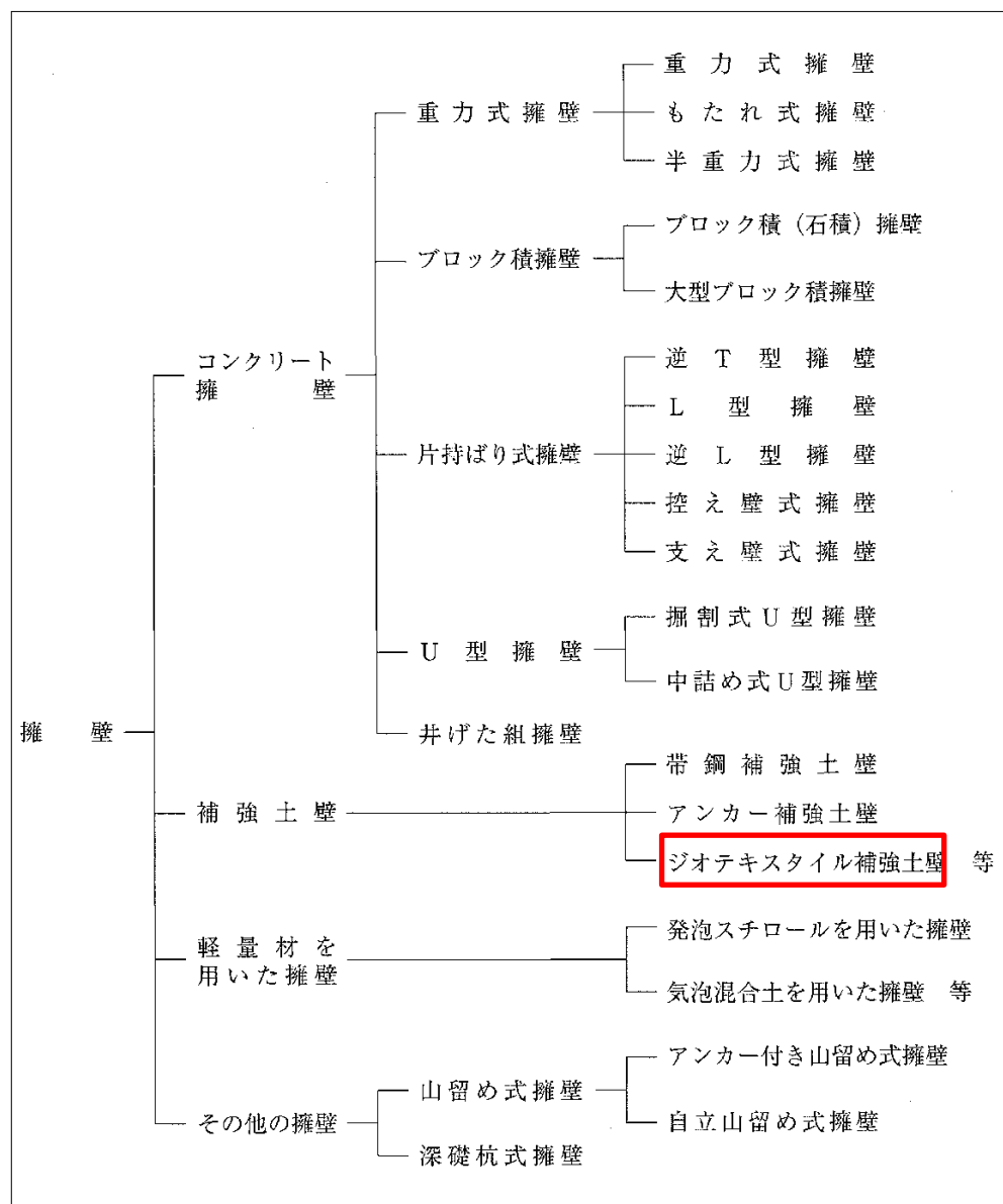
図 3.1 擁壁の分類例
