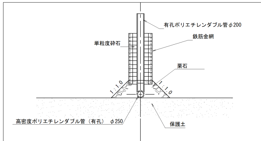
図 3.29 埋立ガス処理施設（堅型ガス抜き管）標準断面図
